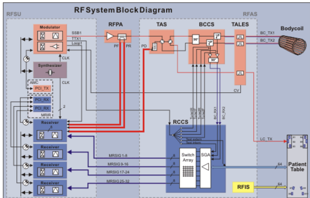
Fig. 353: BCCS_63 - RCCS Loops
