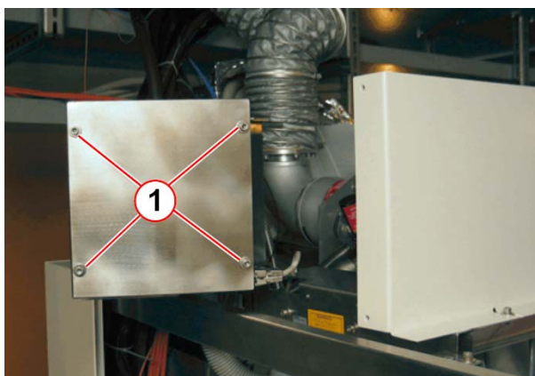
Fig. 475: Patient fan
