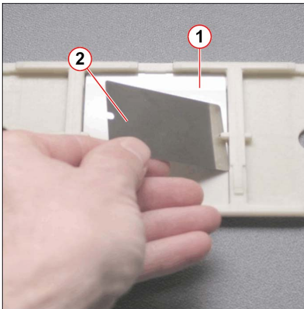
Fig. 305: Shim tray
