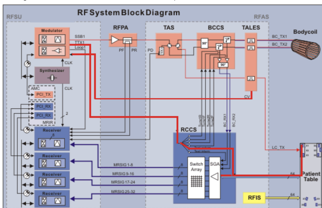
Fig. 351: RCCS interactive test
