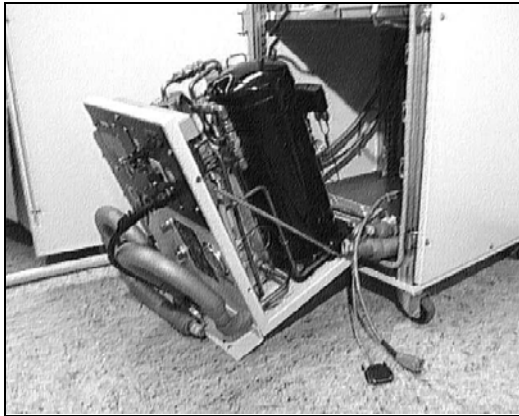
Fig. 501: Cool pack
