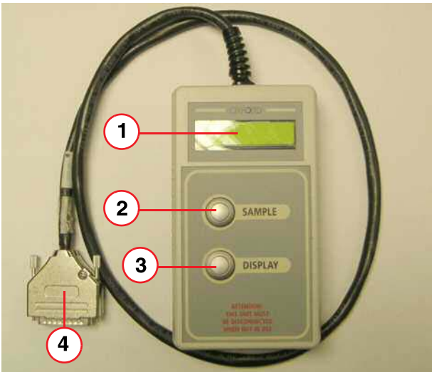
Fig. 457: MSUP- Display Unit
