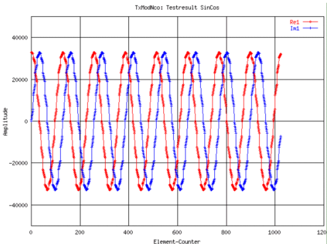
Fig. 330: Complex sine function (TxModNco)
