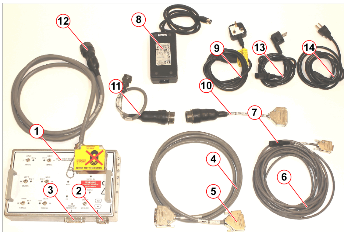
Fig. 456: ERDU Test Load Kit
