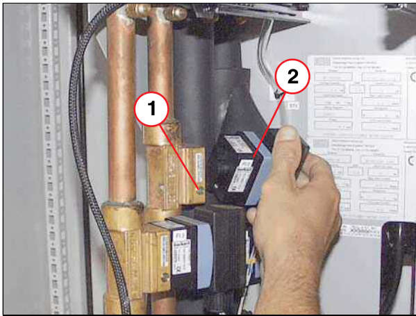
Fig. 482: Flow meter
