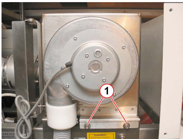
Fig. 474: Patient fan
