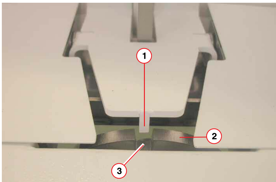
Fig. 448: Trolley Pos. 1 Nib Pos. 2 Disk Pos. 3 Slot
